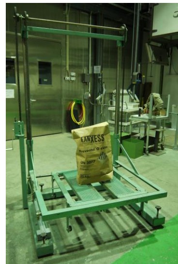
Abb. 20: Fallposition "auf den Sackboden"
