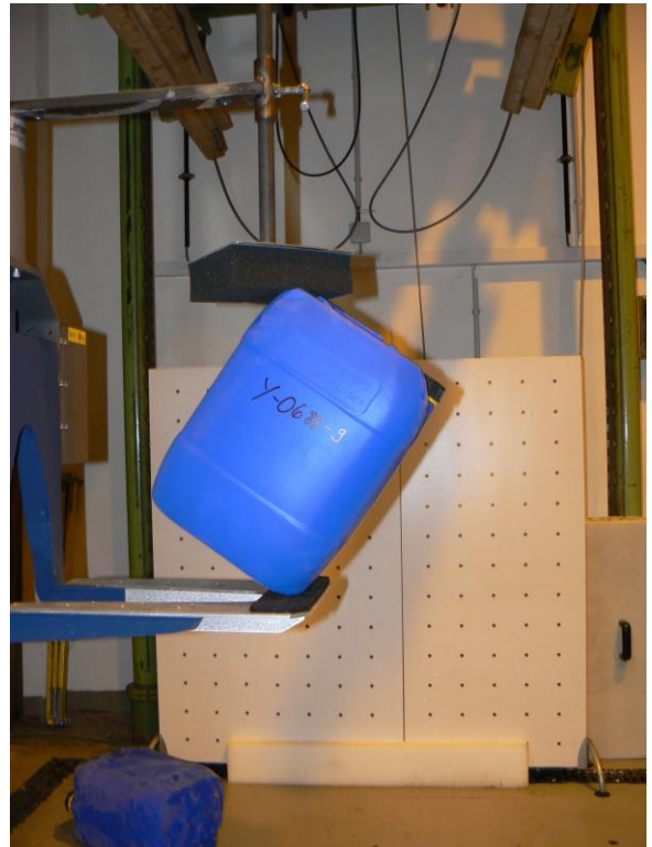
Abb. 11: Kanister diagonal auf Bodenkante
